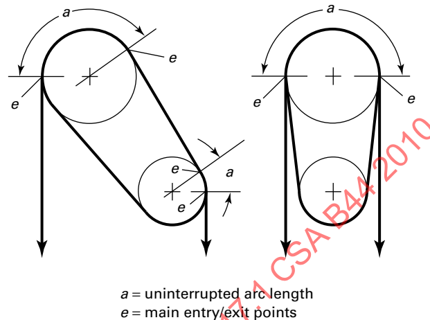
Fig. 8.4.3.1.3 Arc of Contact
