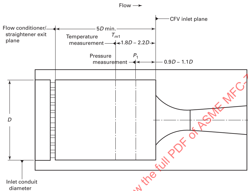
Fig. 7.1-1 Inlet Conduit Schematic
