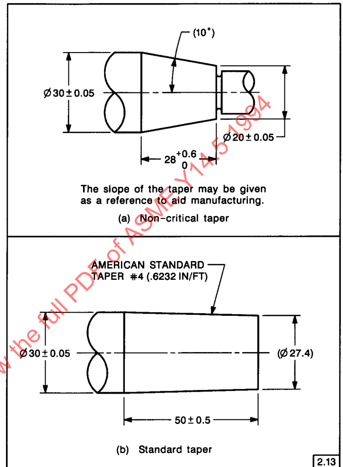
FIG. 2-16 SPECIFYING TAPERS
