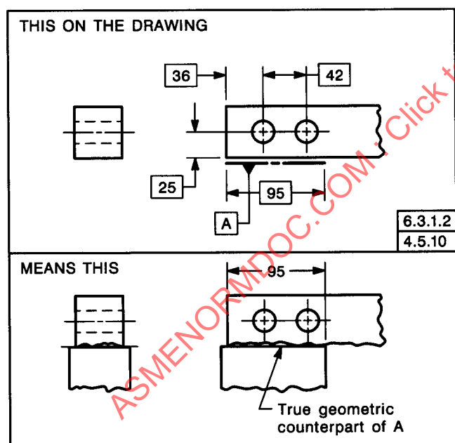
FIG. 4-23 PARTIAL DATUM
