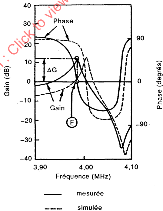
Figure 18 – Caractéristiques gain-phase réellement mesurées et calculées par simulation
