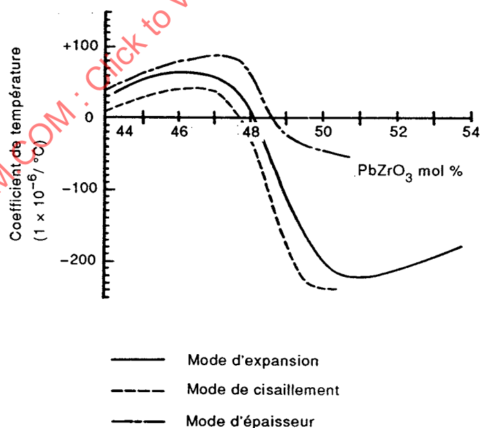
Figure 5 – Caractéristiques du coefficient de température de la fréquence de résonance en fonction du rapport de \text{PbZrO}_3 à \text{PbTiO}_3
