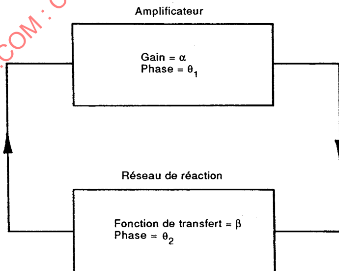
Figure 16 – Principe de fonctionnement d'un circuit oscillateur
