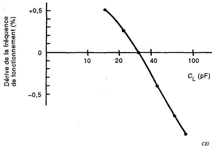
Figure 14 – Exemple de décalage de la fréquence de fonctionnement lorsque la capacité de charge C_L est connectée en parallèle
