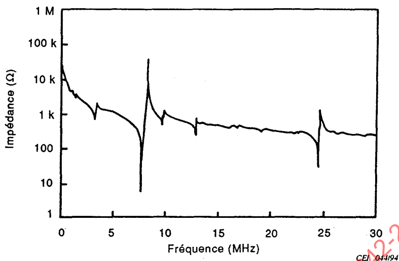
Figure 11 – Caractéristique de l'impédance typique d'un résonateur à céramique piézoélectrique en mode d'expansion d'épaisseur
