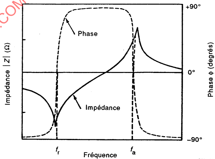
Figure 3 – Variation des caractéristiques de l'impédance et de la phase au voisinage d'une résonance
