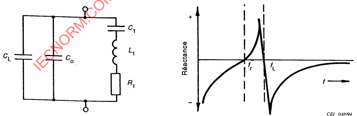
Figure 13c – Résonateur à céramique piézoélectrique connecté en parallèle avec une capacité de charge C_L
