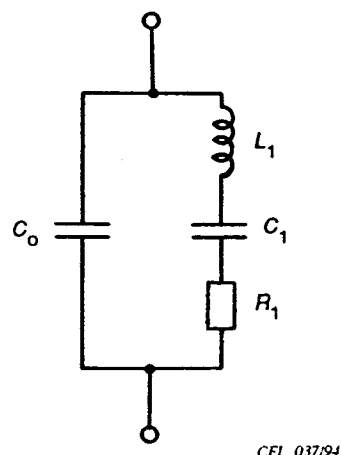
Figure 4 – Circuit équivalent simplifié d'un résonateur à céramique piézoélectrique
