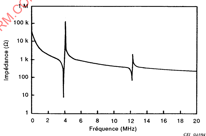
Figure 10 – Caractéristique de l'impédance typique d'un résonateur à céramique piézoélectrique en mode de cisaillement d'épaisseur
