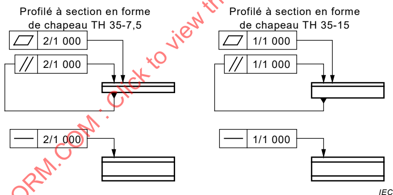
Figure A.4 – Tolérances (TH 35-7,5 et TH 35-15)
