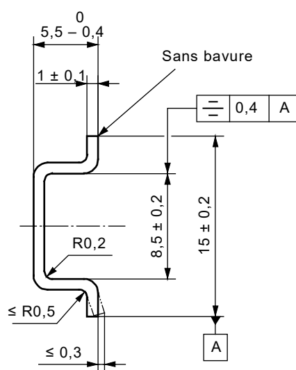
Figure A.1 – Profils à section en forme de chapeau de largeur 15 mm pour fixation d'équipements par encliquetage
