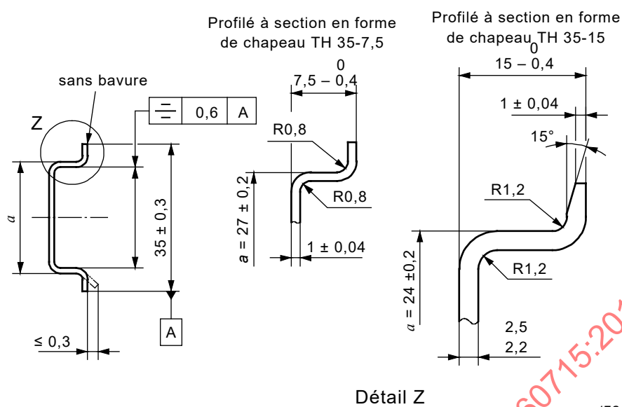
Figure A.3 – Profilés à section en forme de chapeau de largeur 35 mm pour fixation d'équipements par encliquetage
