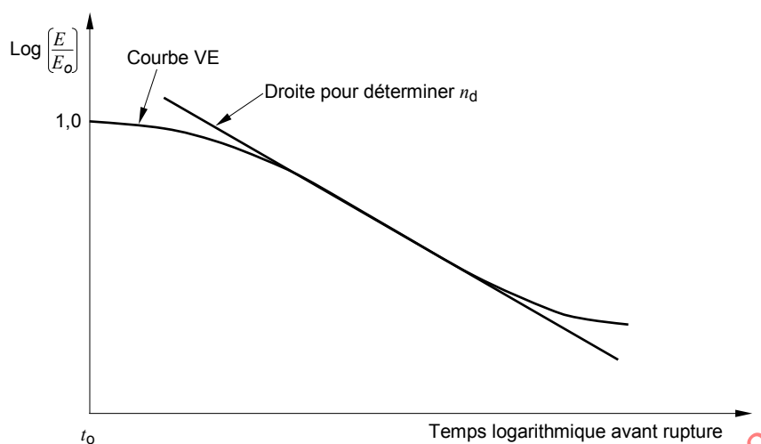
Figure 2 – Détermination du VEC différentiel n_d en un point générique P de la courbe VE
