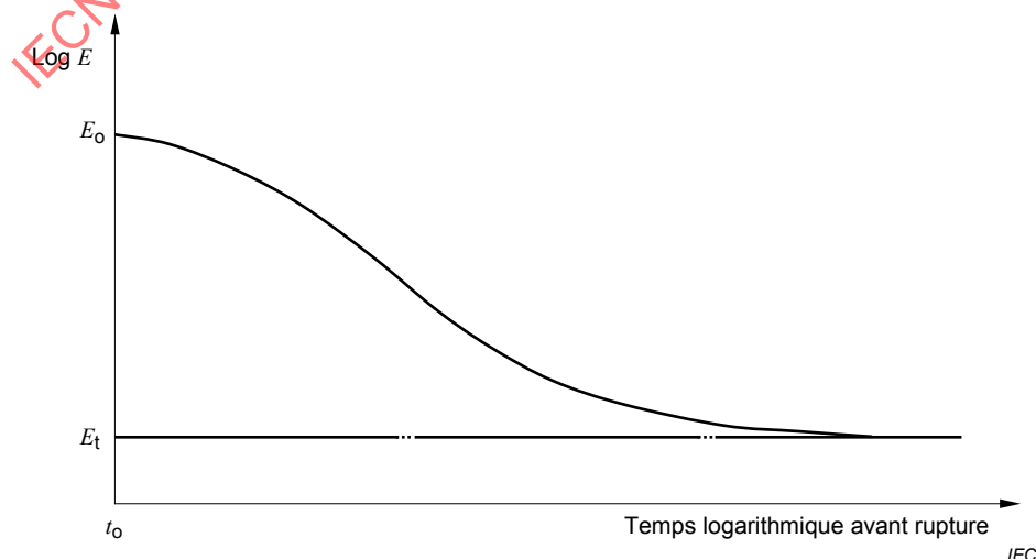
Figure 1 – Courbe d'endurance à la tension générale
