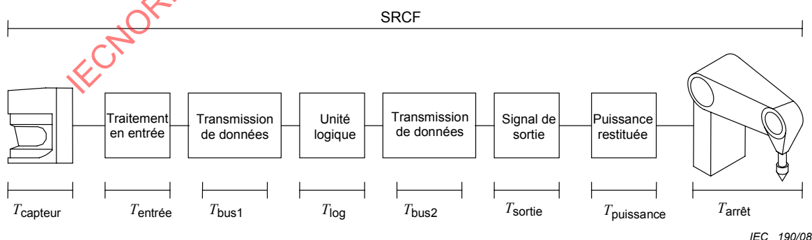
Figure 2 – Composants du temps de réponse du système
