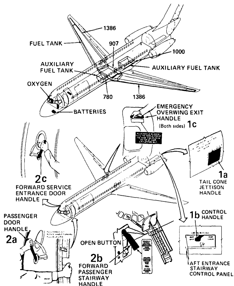
Figure A-23 Douglas DC-9.
